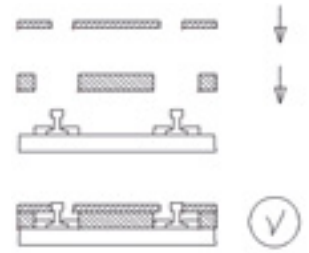
Schematischer Aufbau der N-tram Pflastereinlagen für mini-club®
